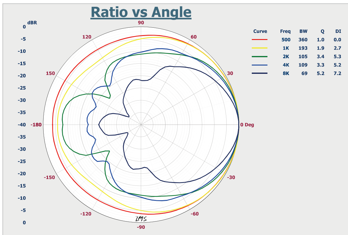
Круговая диаграмма направленности громкоговорителя LPA-20MW
